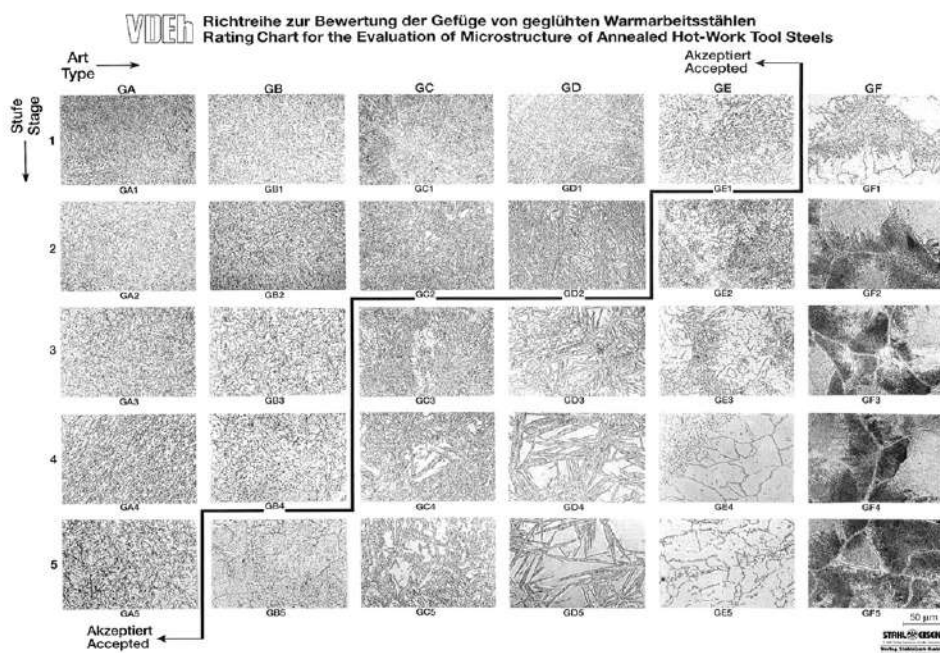
H13系列球化退火组织评级图
